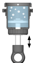
SHOCK OIL INITIAL SETTING 基本セッティング 450cst
