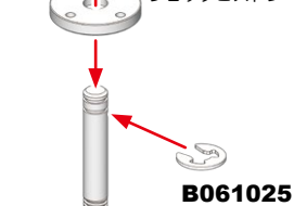
TS055 Shock Shaft 3x18mm ショックシャフト
