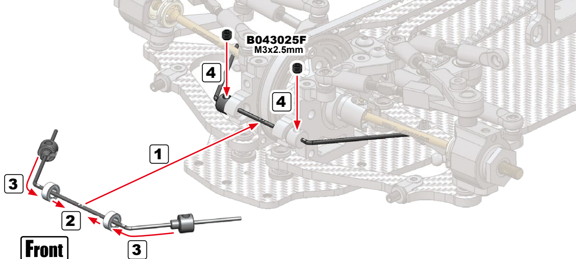
B043025F M3x2.5mm Set Screw (Flat Point) セットスクリュー (平先)
